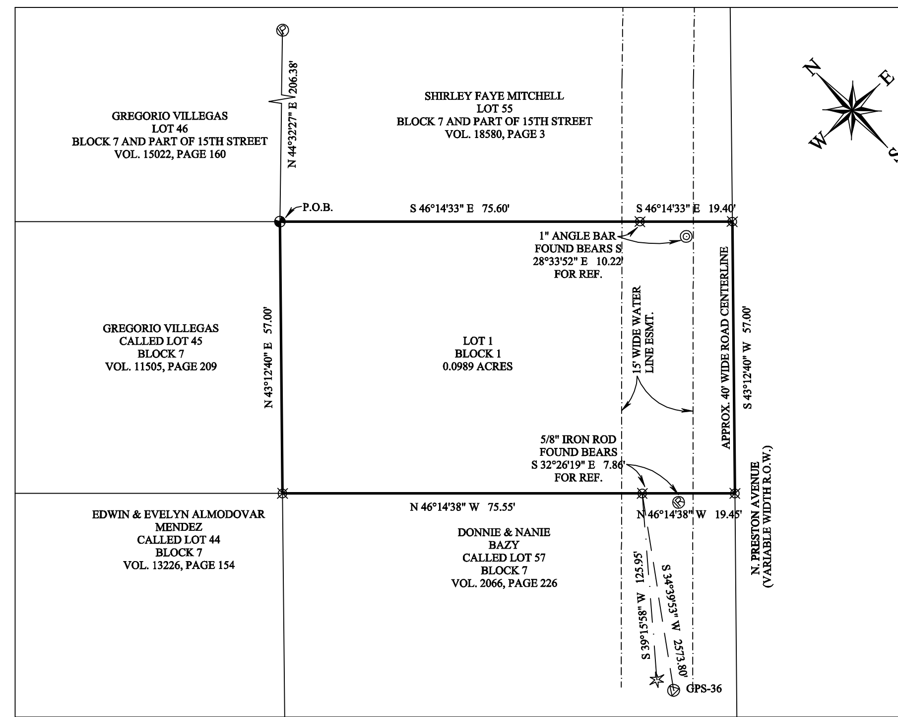
FINAL PLAT
